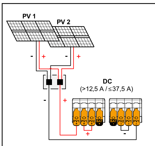
Kombinované vetvy solárneho modulu so súčtovým prúdom ( I_{dcmax} ) väčším ako 12,5 A.
