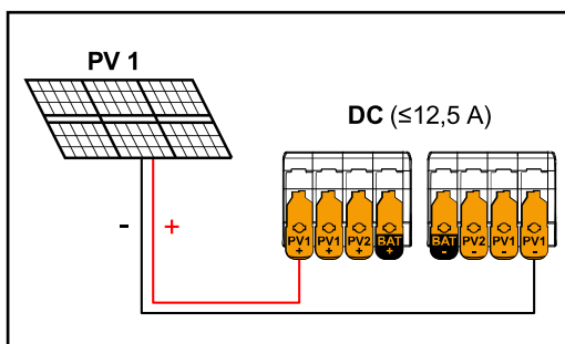
Súčtový prúd ( I_{dcmax} ) menší/rovný 12,5 A.
